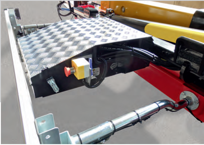
Steuerblock für Funkfernsteuerung
